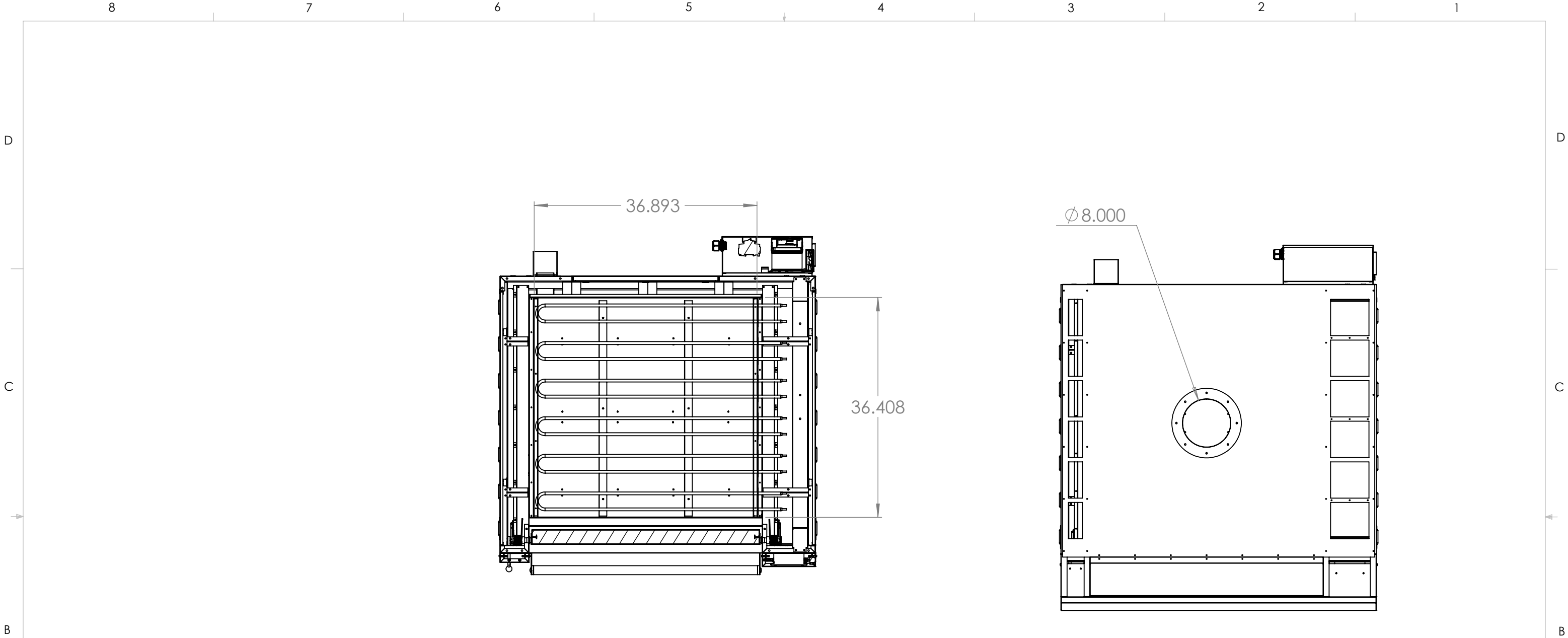
SECTION B-B SCALE 1 : 16
